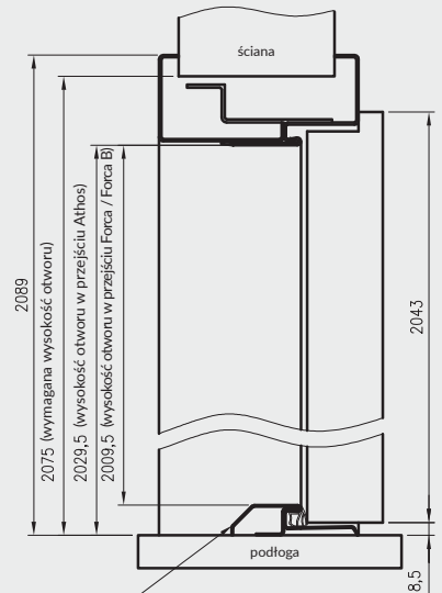
Próg stały (stalowy) do drzwi Forca i Forca B lub uszczelka opadająca w drzwiach Athos
