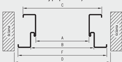
Przekrój poprzeczny
