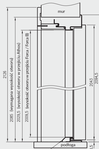
przekrój pionowy
