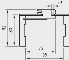
Przekrój ORB 075
