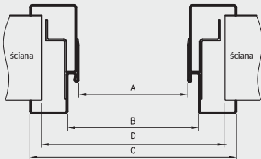
przekrój poziomy ościeżnicy w murze
