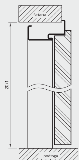
przekrój pionowy alternatywny sposób montażu
