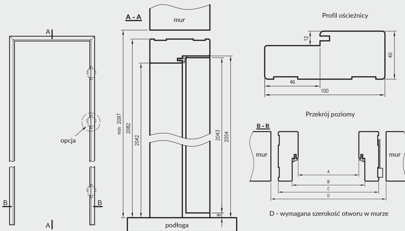
Przekrój pionowy drzwi bezprzylgowych OPB
