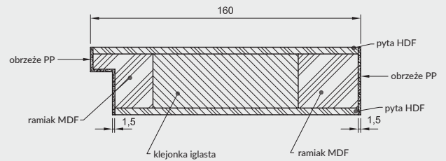
PRZEKRÓJ RAMIAKA PIONOWEGO
