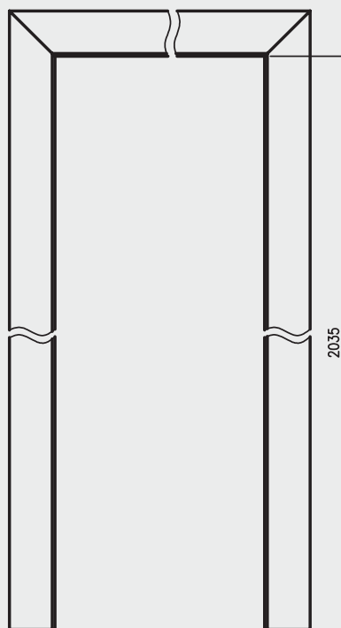
Przekrój pionowy tunelu regulowanego z ką. T80
