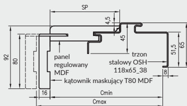
profil ościeżnicy
