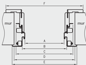
przekrój poziomy ościeżnicy w murze
