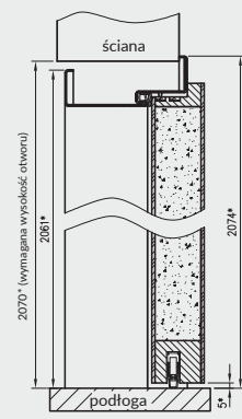
Przekrój pionowy przy montażu na zaprawę murarską
