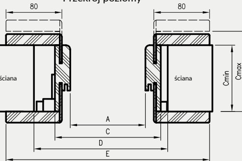
D - wymagana szerokość otworu w murze
