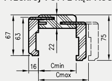
Przekrój TUN z ką. K63
