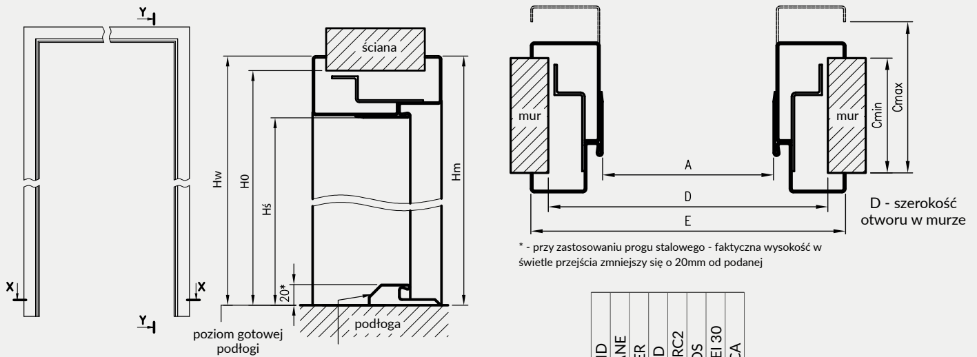
Wymiary OSR STAND dla drzwi dwuskrzydłowych
