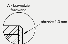
Przekrój ramiaka skrzydła bezprzylgowego
